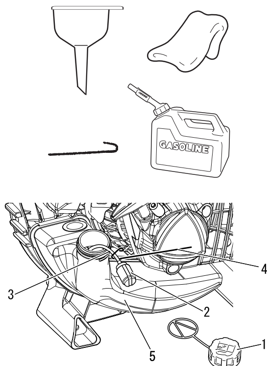
1. Bouchon du réservoir de carburant 2. Filtre à carburant 3. Tuyau d'alimentation de carburant 4. Crochet du tuyau d'alimentation 5. Réservoir de carburant
