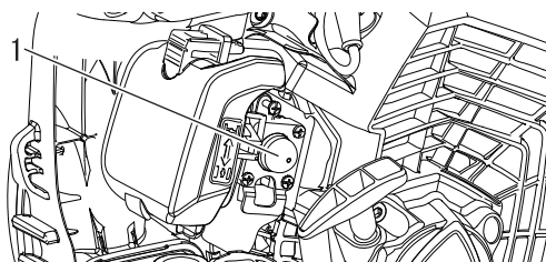
1. Kraftstoffpumpe
