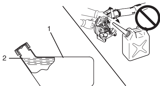
1. Réservoir de carburant 2. Épaulement
