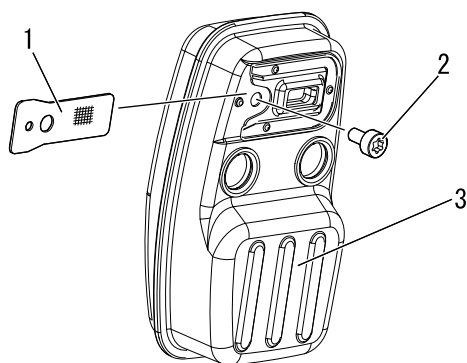
1. Funkenschutzsieb
