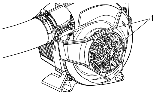
1. Gehäuse-Abdeckung
