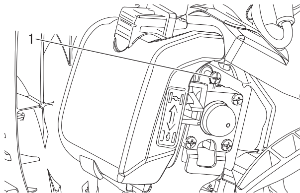
1. Schraube
