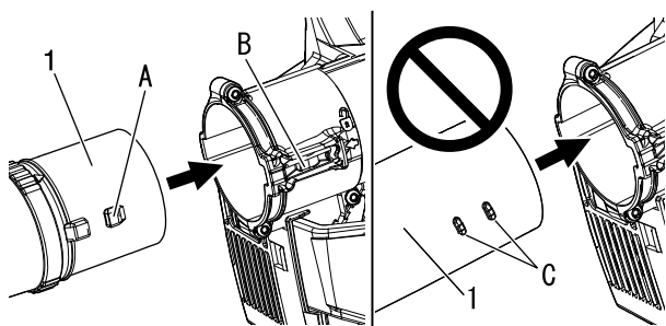
1. Rohr
