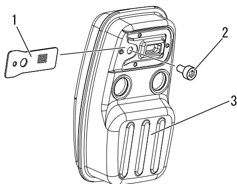
1. Pantalla protectora del apaga chispas 3. Silenciador
