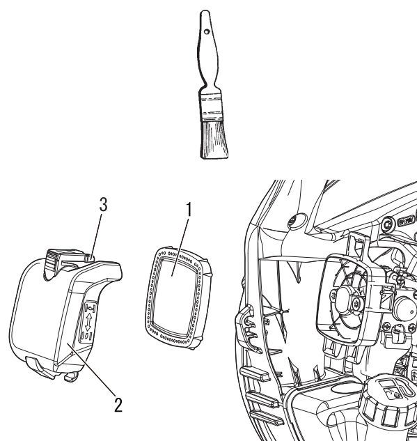
1. Filtre à air 2. Couvercle du filtre à air 3. Loquet du filtre à air
