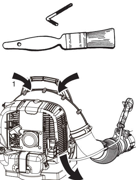
1. Admission d'air
