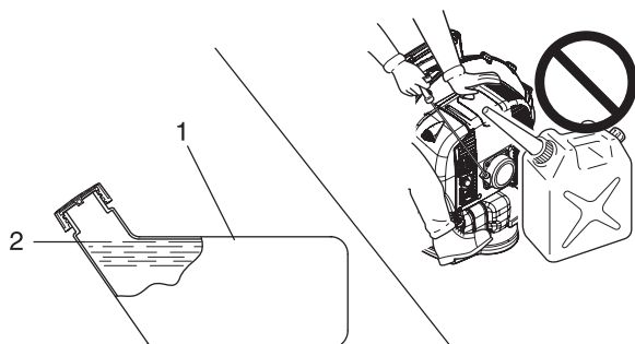
1. Kraftstofftank
