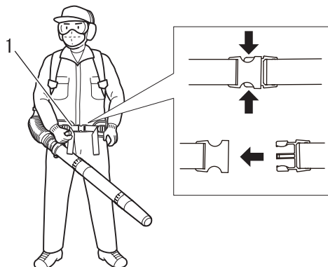
1. Ceinture dorsale
