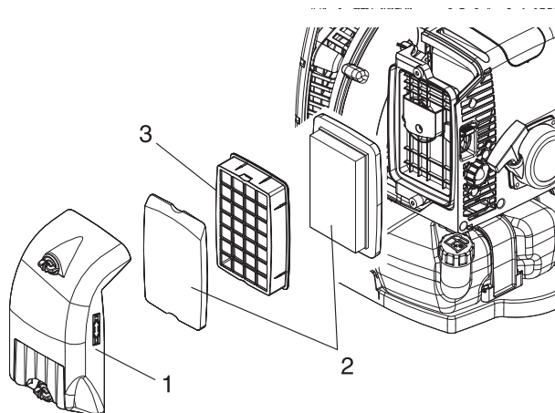
1. Luftfilterabdeckung 3. Laubsieb
