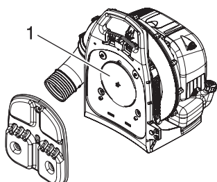
1. Ansaugabdeckung
